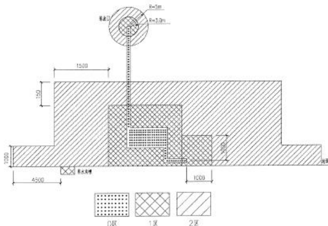
图3-4 三次油气回收装置爆炸危险区域划分 (单位: mm)
