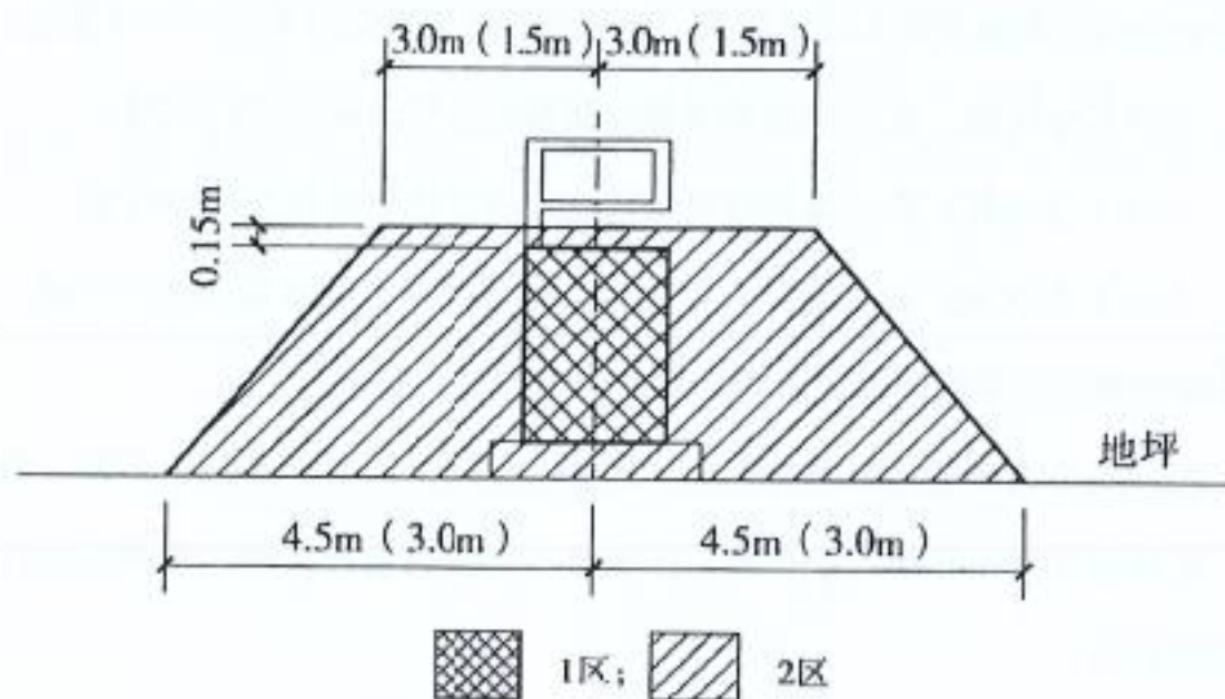
图 3-1 汽油加油机爆炸危险区域划分
